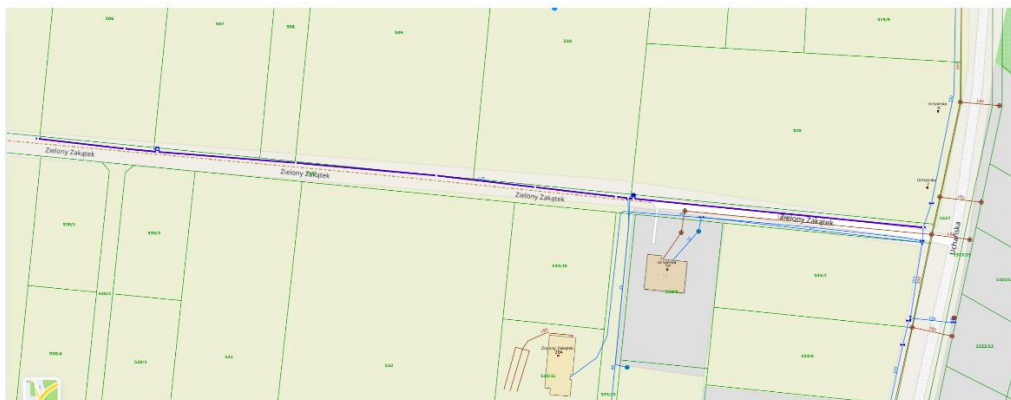
Wybudowany odcinek sieci wodociągowej w ulicy Zielony Zakątek, etap A-B
